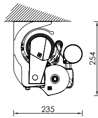
Montaggio a soffitto con staffa universale Ceiling installation with universal bracket
