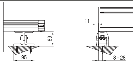
supporto guida regolabile e inclinabile - Inclinal and adjustable guide support
