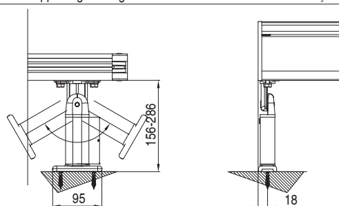
supporto guida regolabile e inclinabile - Inclinal and adjustable guide support
