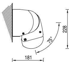
Installazione a parete 75°
