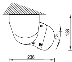
Installazione a soffitto 15°
