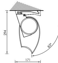
Montaggio a soffitto 85° Ceiling installation 85°
