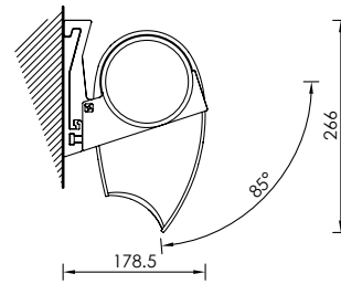
Montaggio a parete 85° Wall installation 85°
